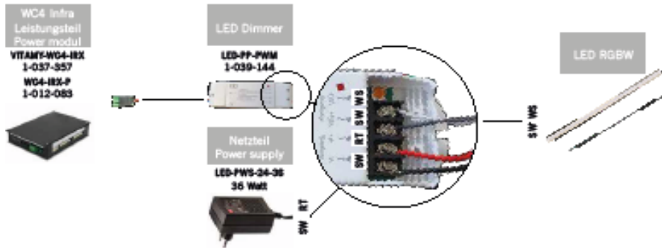
Abb. 27: Verbinden des LED RGBW mit der Steuerung
