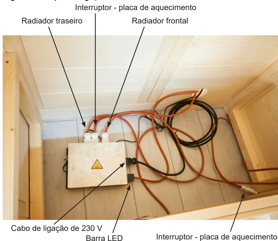
Fig. 25: Exemplo de ligação
