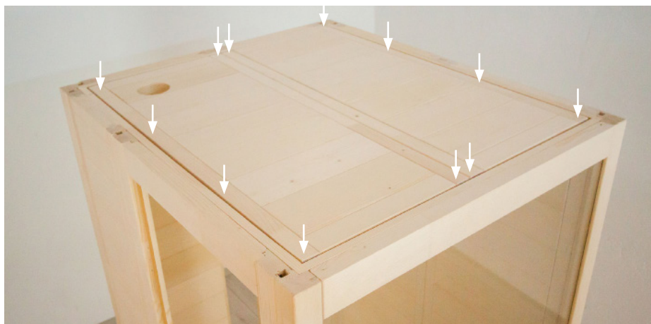
Fig. 15: Fixação dos elementos de teto
